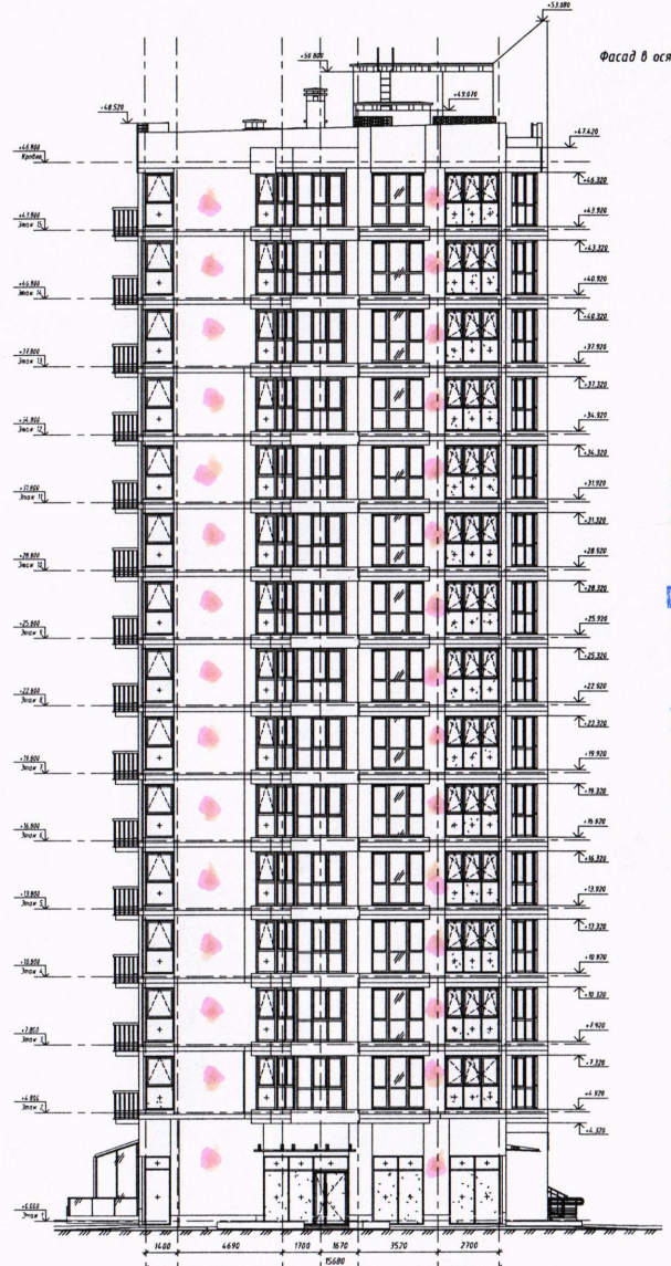
Фасад в осях А-Л
