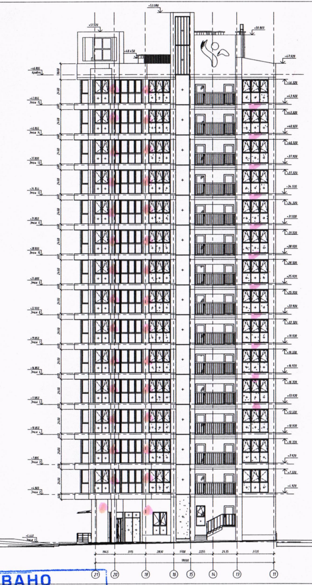
Фасад в осях 21-12
