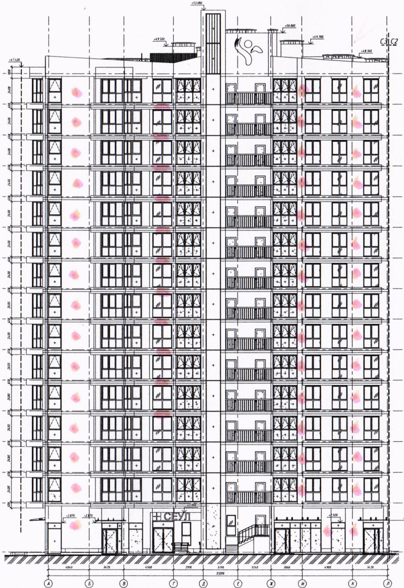
Фасад в осях А-Л
